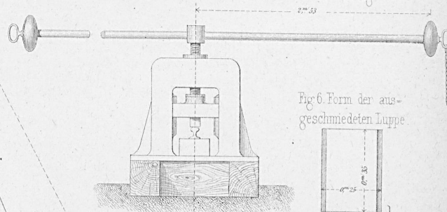
Fig. 3. Schraubenpresse zur Probe auf Textur und Schweißung.
