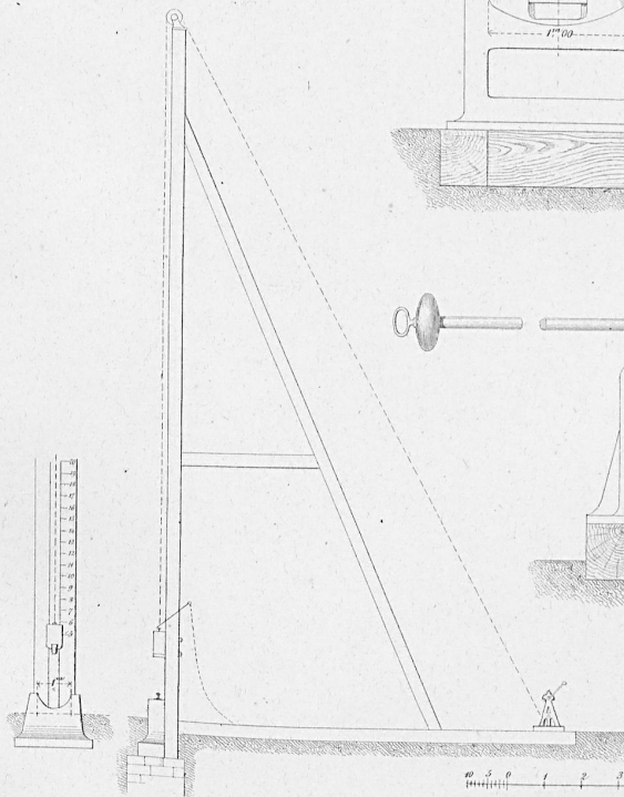
Fig. 4. Fallvorrichtung zur Probe auf die Bruchsicherheit.
