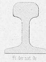
Fig. 5. Vignoles Schiene der Oesterr. Südbahn.
