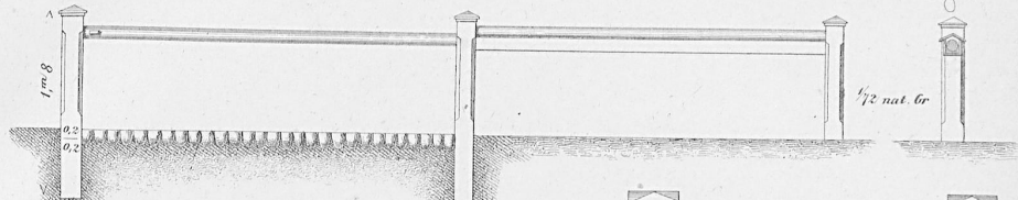
Fig. 1. Schiebe-Barrière für Wegeübergänge von 3 m 6-5 m 0 Weite.
