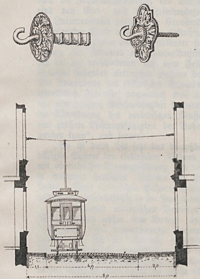
Strassenprofil (Braunstrasse in Lübeck) und Rosetten zur Befestigung der Leitung an den Häusern.
