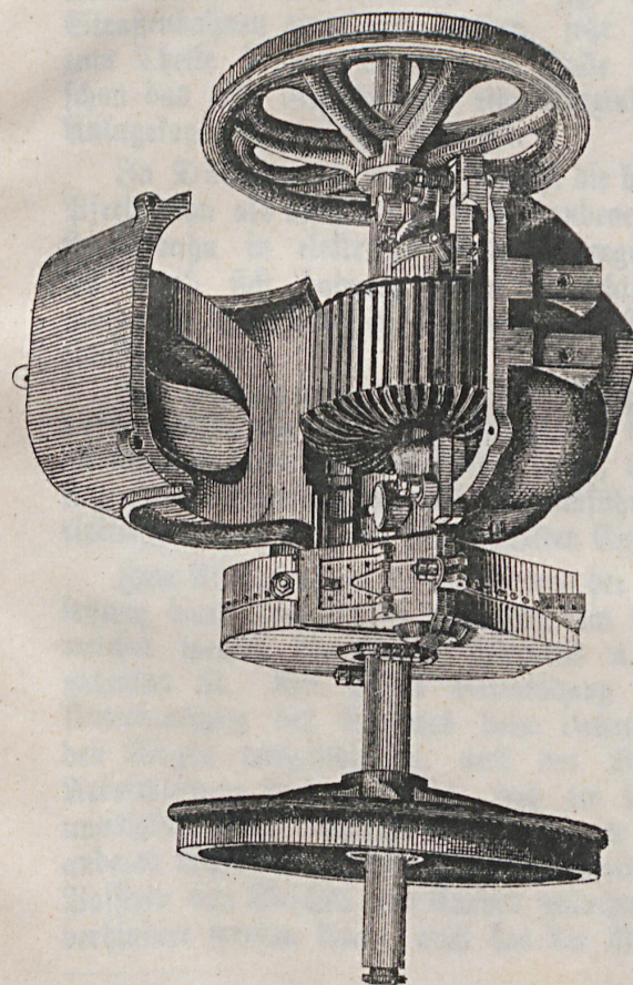
Motor am Wagen (aufgeklappt.)
