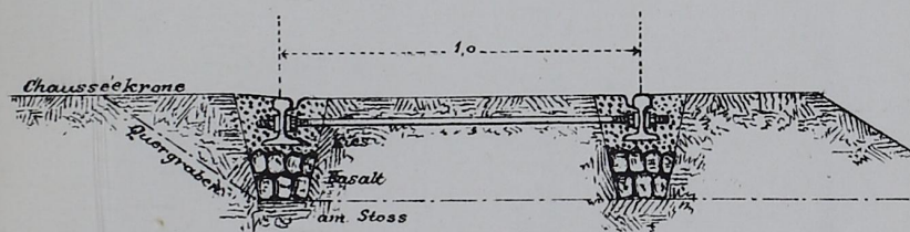
Querprofil .
