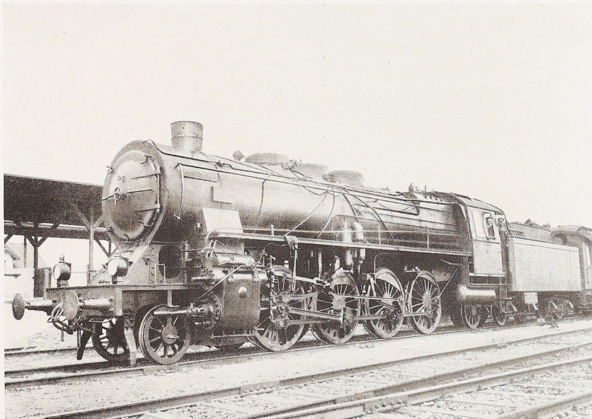
Bild 18. Die 11 000. Borsig-Lokomotive (Bild 19) mit Meßapparaten auf der Probefahrt. Druckstock: A. Borsig, Berlin-Tegel.
