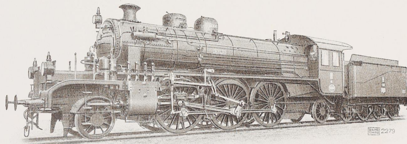
Bild 34. 1 C 1-Zweizylinder-Heißdampf-Schnellzuglokomotive mit Lentz-Ventilsteuerung der ehemaligen Oldenburgischen Staatsbahnen. Als Fabriknummer 8000 erbaut von der Hanomag, Hannover-Linden. Druckstock: Hanomag, Hannover-Linden.
