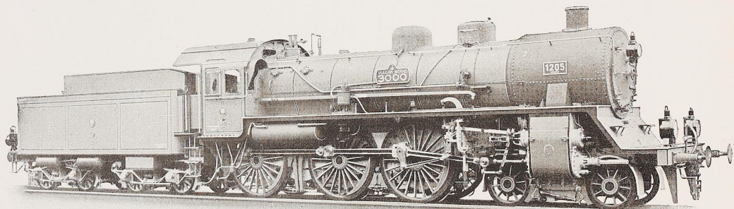
Bild 35. 2 C-Dreizylinder-Heißdampf-Schnellzuglokomotive Gattung S10 2 der ehemaligen Preußisch-Hessischen Staatsbahnen. Als Fabriknummer 3000 erbaut von den Vulcan-Werken A. G., Hamburg und Stettin. Druckstock: Vulcan-Werke, Stettin.
