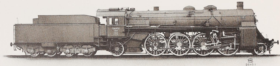
Bild 33. 1 D 1-Dreizylinder-Heißdampf-Schnellzuglokomotive (Reihe XVIII H) der ehemaligen Sächsischen Staatsbahnen. Als Fabriknummer 4000 erbaut von der Sächsischen Maschinenfabrik vorm. R. Hartmann A.-G., Chemnitz. Druckstock: Sächsische Maschinenfabrik vorm. R. Hartmann A.-G., Chemnitz.
