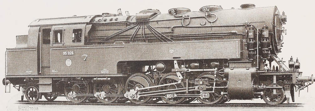
Bild 58. 1 E 1-Zweizylinder-Heißdampf-Güterzug-Tenderlokomotive Gattung T 20 der Deutschen Reichsbahn. Erbaut von der Hanomag, Hannover-Linden. Druckstock: Hanomag, Hannover-Linden
