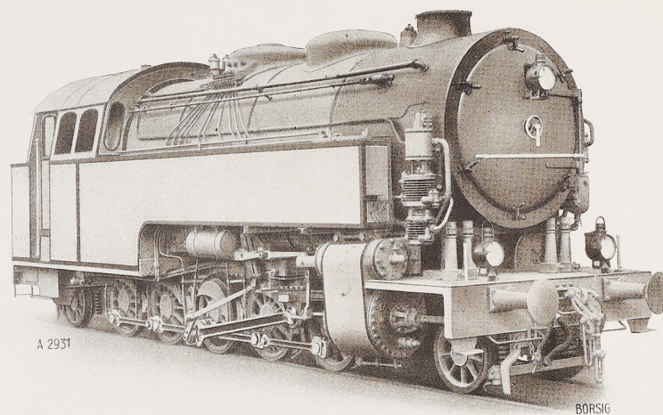
Bild 57. 1 E 1-Zweizylinder-Heißdampf-Güterzug-Tenderlokomotive der Halberstadt—Blankenburger Eisenbahngesellschaft. Erbaut von A. Borsig, Berlin-Tegel. Druckstock: A. Borsig, Berlin-Tegel.
