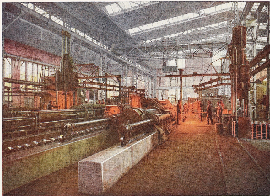
Bild XII. Ein Blick in die Werkhallen der Maschinenbau-Anstalt Humboldt, Köln-Kalk: Hydraulische Horizontal-Pressenanlage.
