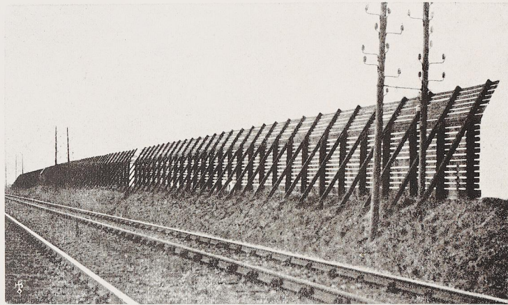
Bild 334. Die Wächter des eisernen Pfades: Schneezaun an einer Hauptstrecke der Französischen Staatsbahn.
