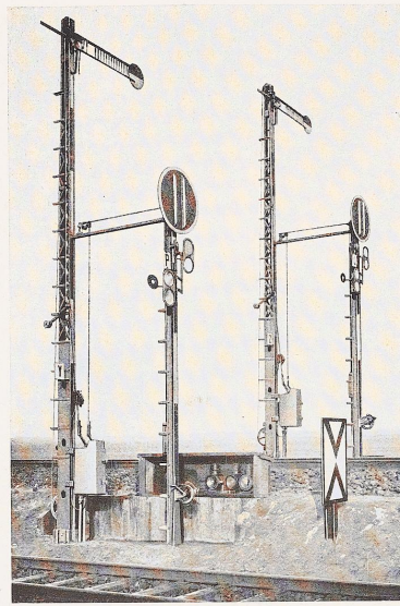
Bild 342. Die Wächter des eisernen Pfades: Von einer einzigen Kraftquelle aus angetriebene Vor- und Hauptsignale verschiedener Streckenabschnitte (Bahnhof Wustermark). Ausgeführt von Siemens & Halske A.-G., Blockwerk, Siemensstadt bei Berlin.
