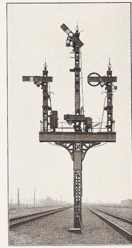
Bild 343. Die Wächter des eisernen Pfades: Auslegersignal der Belgischen Staatsbahnen. Ausgeführt von Siemens & Halske A.-G., Blockwerk, Siemensstadt bei Berlin.
