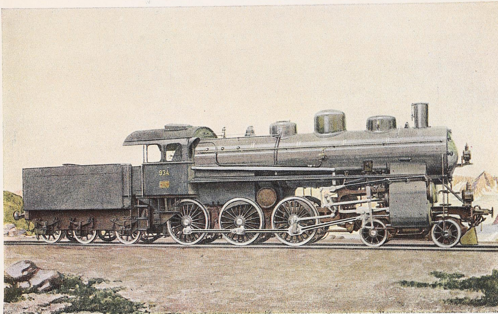
Bild XVIII. 2 C-Vierzylinder-Verbund-Gebirgslokomotive der Schweizer Bundesbahnen (Gotthardstrecke). Erbaut von J. A. Maffei, München. Farbplatten: J. A. Maffei, München.
