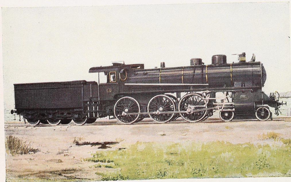
Bild XXI. 2 C-Vierzylinder-Verbund-Schnellzuglokomotive der Portugiesischen Staatsbahnen (Spurweite 1665 mm). Erbaut von J. A. Maffei, München. Farbplatten: J. A. Maffei, München.
