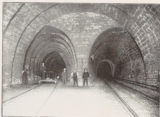
Bild 511. Simplonbahn: Simplontunnel (Bild 499). Ausweich- und Signalstation in der Tunnelmitte, die Landesgrenze zwischen der Schweiz und Italien. Zusammentreffen beider Einzelstollen in einem einzigen Hauptstollen. Druckstock: Schweizer Bundesbahnen, Bern.
