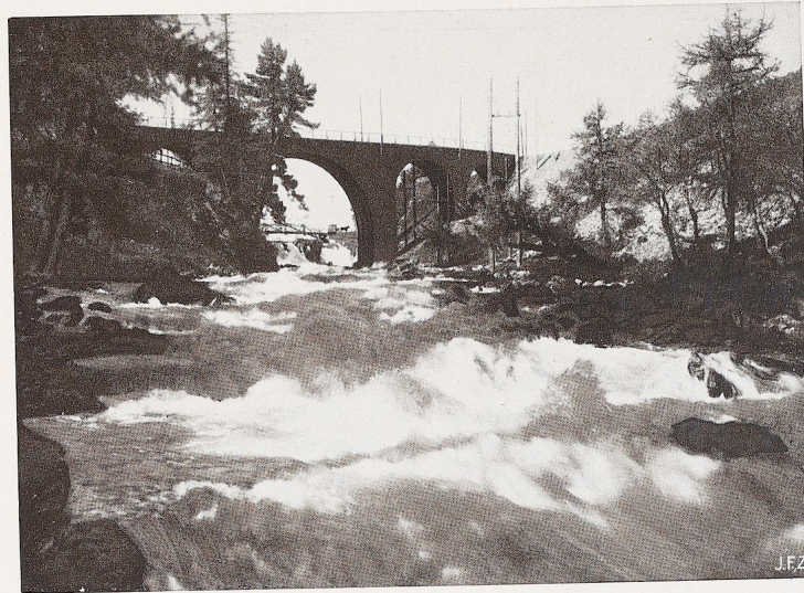
Bild 576. Berninabahn: Nordrampe. Inn-Viadukt bei St. Moritz. (Spannweite der Mittelöffnung 18 m, der linken und beiden rechten Seitenöffnungen je 10 m). Im Hintergrund der Innfall. Druckstock: Berninabahn, Poschiavo.
