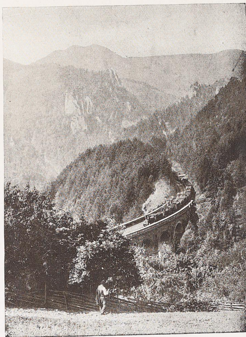
Bild 597. Semmeringbahn: Nordrampe. Güterzug auf dem zweistöckigen Viadukt über den Wagnergraben von Bild 599. (Spannweite der fünf unteren segmentförmigen Gewölbe je 9,48 m, der neun oberen halbkreisförmigen Gewölbe je 12,3 m, Fahrbahnhöhe 39 m, Gesamtlänge 142 m). Druckstock: Landesverband für Fremdenverkehr in Niederösterreich, Wien.
