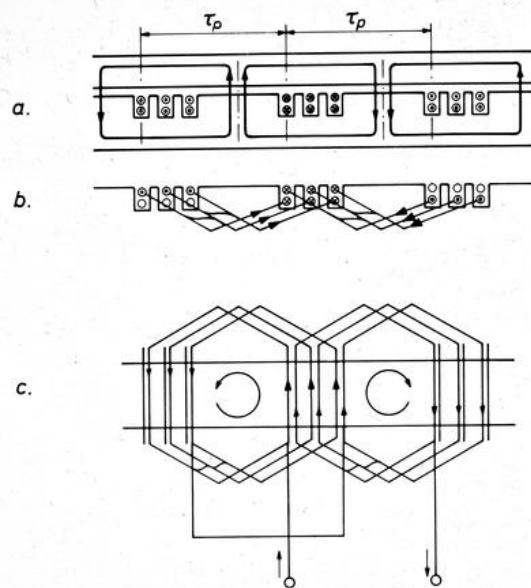
EW THD Entstehung eines Wicklungsstranges einer ungesehenen Zweischichtwicklung für q=3 1/4.4
