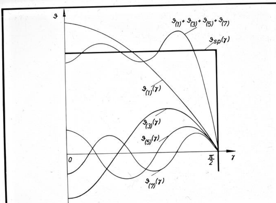
EW Durchflutungsverteilung i_{sp}(\gamma) einer ungesehnten Einzelzspule. Zerlegung in die ersten sieben Harmonischen
