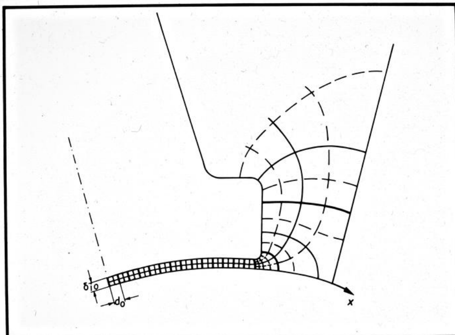
EW THD Feldbild zur Ermittlung der Induktions- verteilung an der Läuferoberfläche 1/5.18
