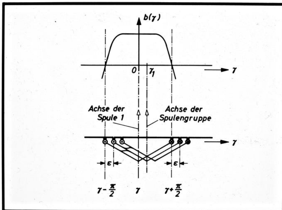
EW Zur Induzierung einer Spulengruppe THD je Polpaar (Einschichtwicklung)
