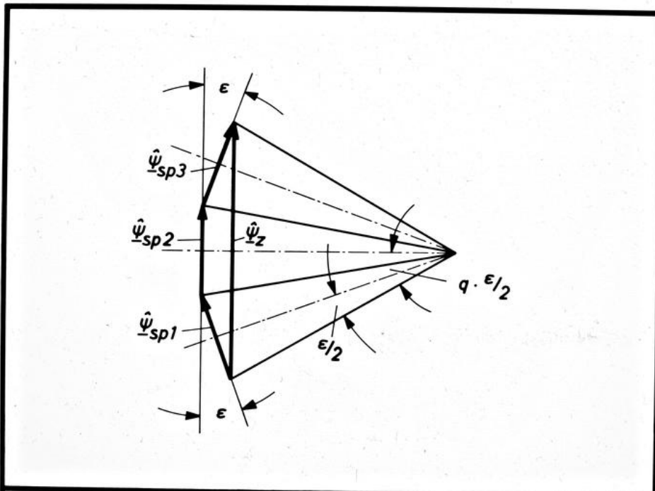
EW Zonenfaktor für die Grundwelle THD der Flußverkettung
