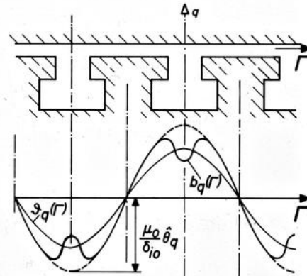
b) Querkomponente
