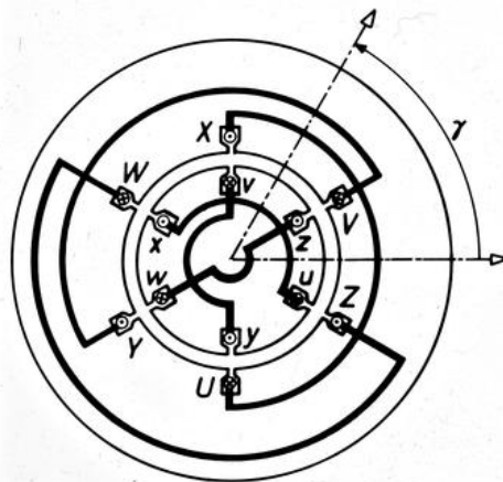
a) Querschnittsdarstellung
