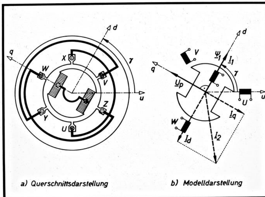
EW Grundsätzlicher Aufbau und Modell der THD dreisträngigen Schenkelpol - Synchronmaschine
