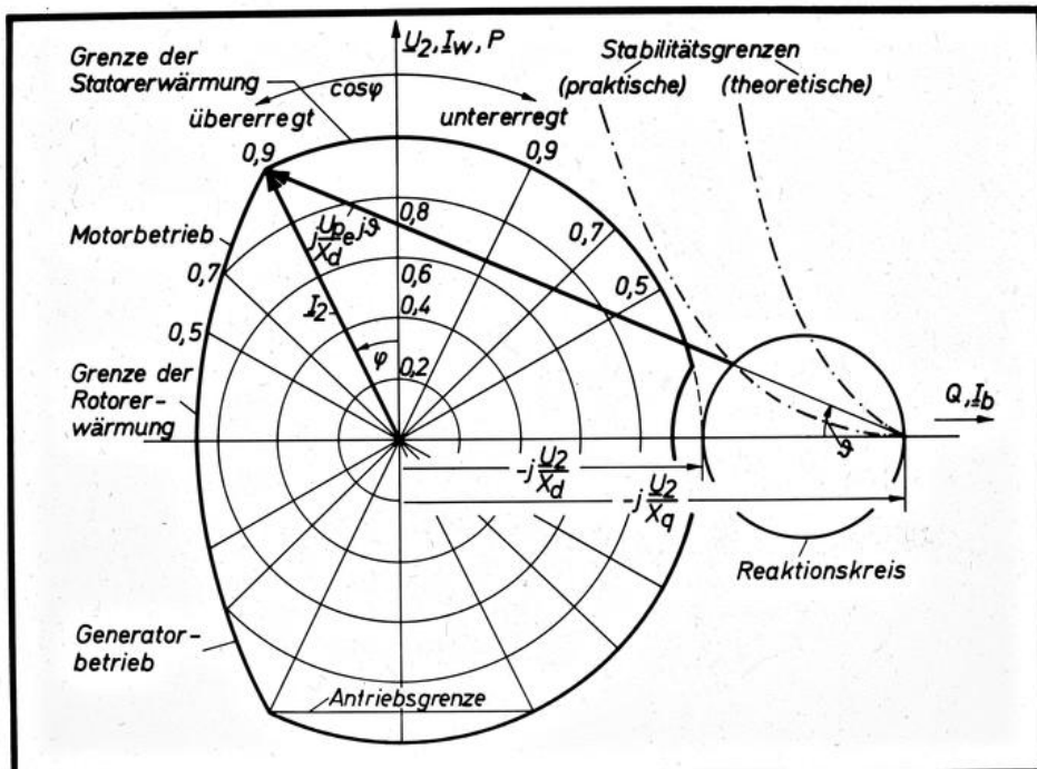
EW Vollständiges Strom- und Leistungsdiagramm THD der Schenkelpolmaschine
