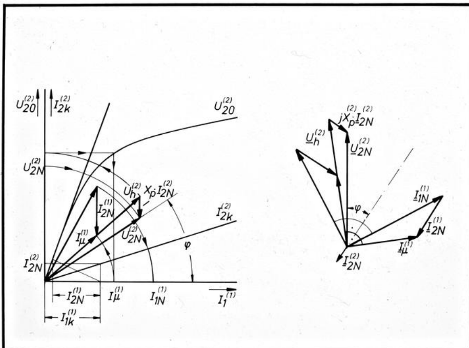
EW THD Bestimmung der Erregung einer Vollpol - Synchronmaschine (Generator übererregt)
