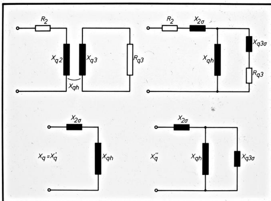
EW THD Ersatzschaltungen und Reaktanzen der Synchronmaschine in der Querachse
