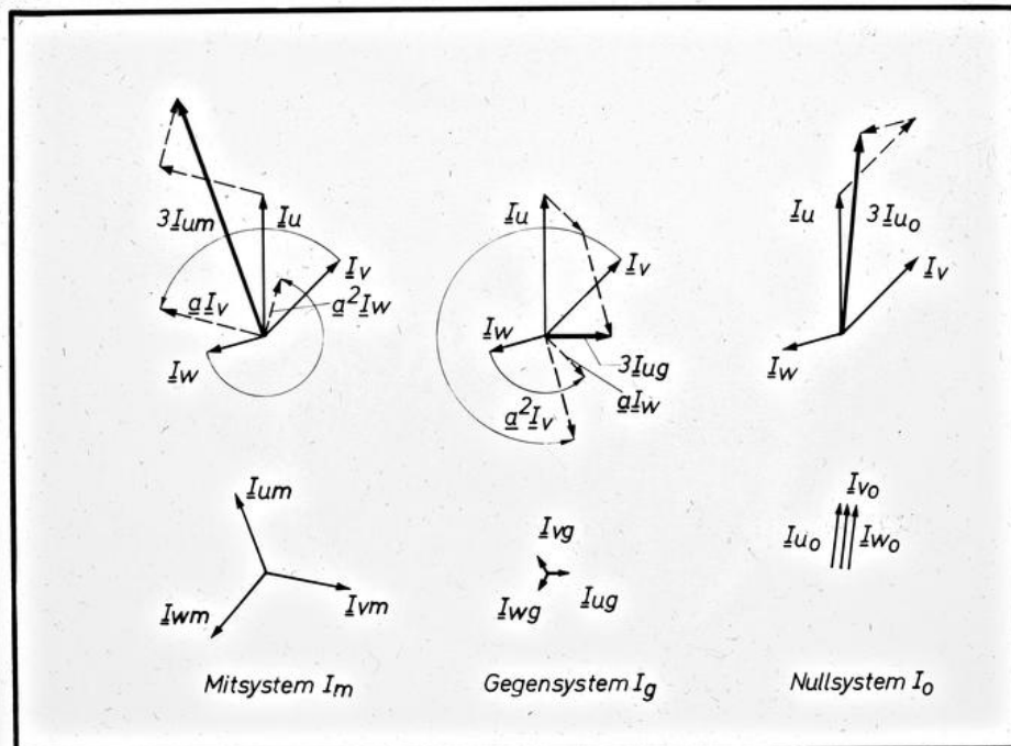
EW Zerlegung eines unsymmetrischen Drehstromsystems THD in symmetrische Komponenten
