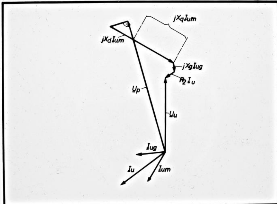
EW THD Zeigerdiagramm für den Strang u der unsymmetrisch belasteten Synchronmaschine
