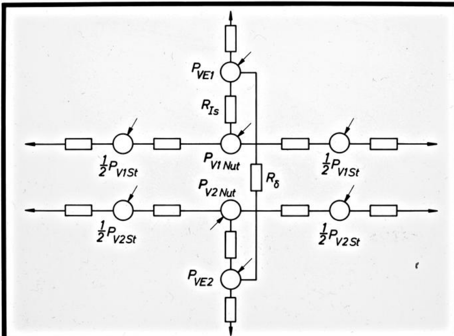
EW Ersatzschaltbild für den Wärmestrom THD (zur Wärmequellennetzmethode)
