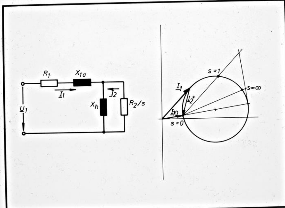
EW Angenähertes Ersatzschaltbild u. Stromortskurve THD eines asynchronen Linearmotors großer Polzahl 2/4.18
