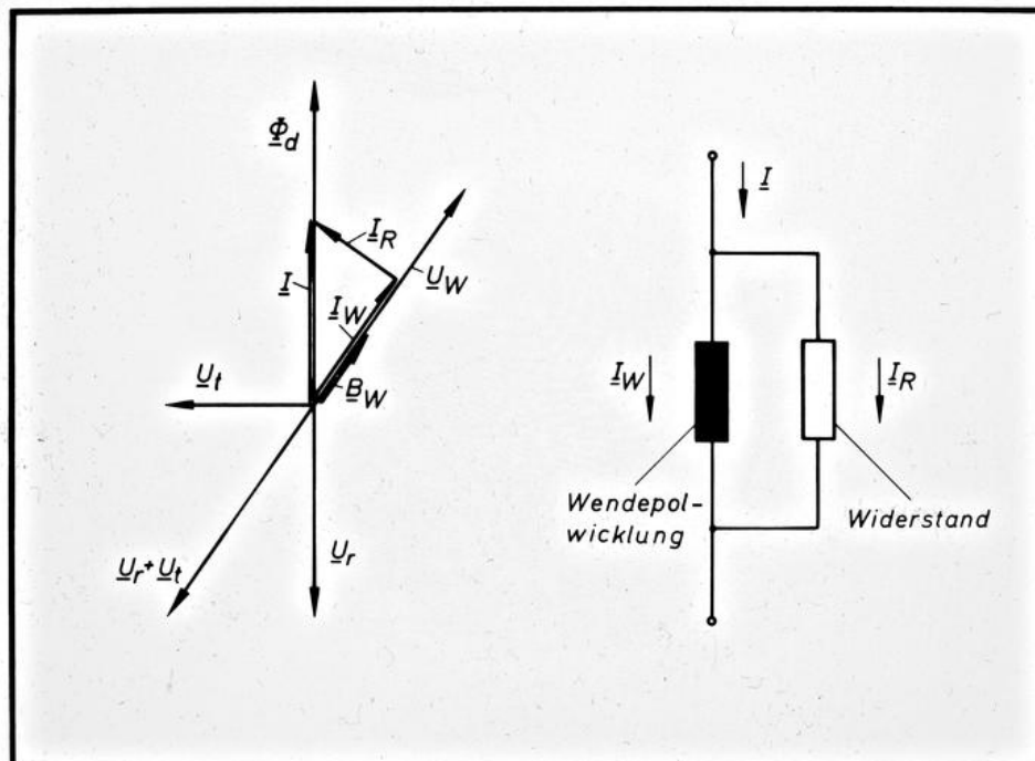
EW Zeigerdiagramm für die kommutierenden 2/5.6 THD Spulen und Hilfsschaltung
