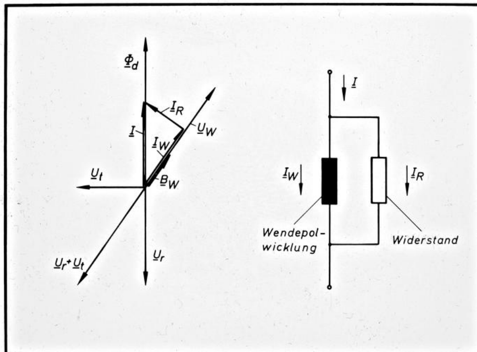
EW THD Zeigerdiagramm für die kommutierenden Spulen und Hilfsschaltung 2/5.6
