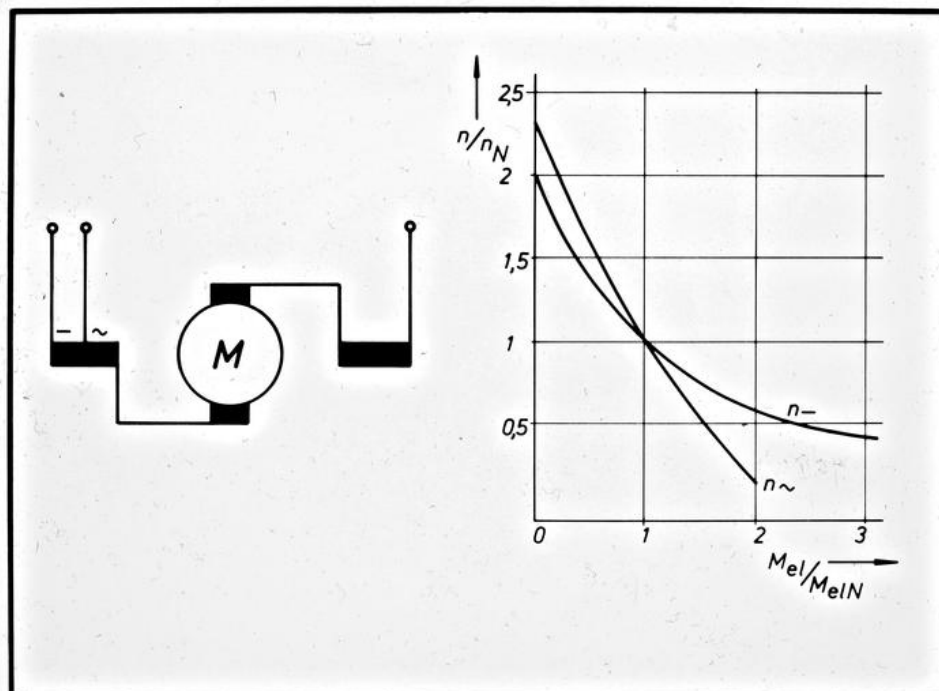
EW Schaltung und Kennlinie des Universalmotors THD für Betrieb mit Gleich- und Wechselstrom 2/5.8
