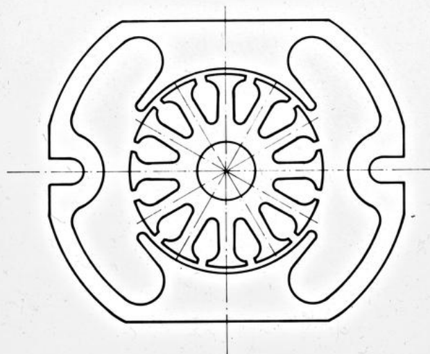
EW THD Ständer - u. Läuferblechschnitt eines Universalmotors 2/5.9
