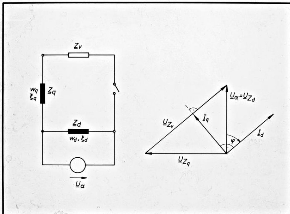
EW Der zweisträngige Einphasen-Asynchronmotor 2/4.6 THD mit Vorimpedanz
