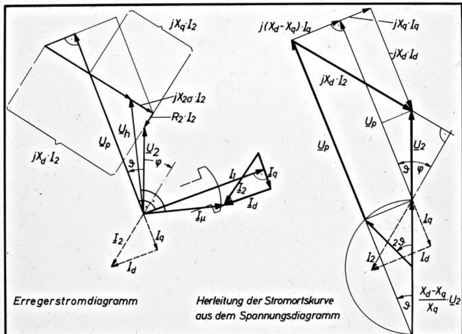
EW Zeigerdiagramme der Synchron-Schenkelpol- THD maschine, Generatorbetrieb, übererregt
