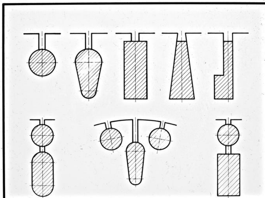
EW THD Stabformen von Einfach- und Doppelkäfigen
