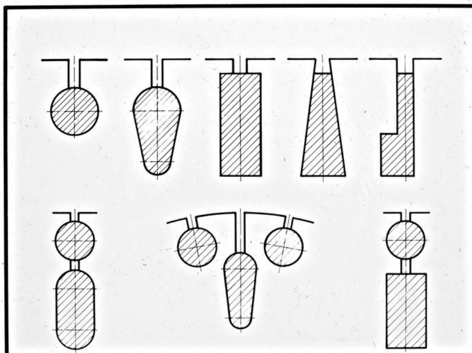
EW Stabformen von Einfach- und THD Doppelkäfigen
