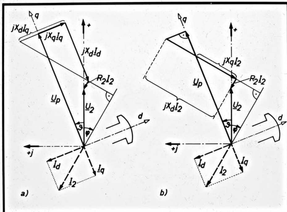
EW Zeigerdiagramm der Synchron-Schenkelpolmaschine, THD Generatorbetrieb, übererregt
