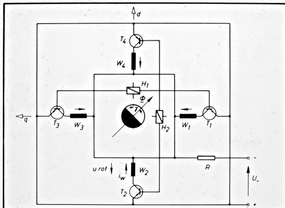
EW THD Wirkschlupfplan für hallgesteuerten Elektronikmotor. 2/5.13
