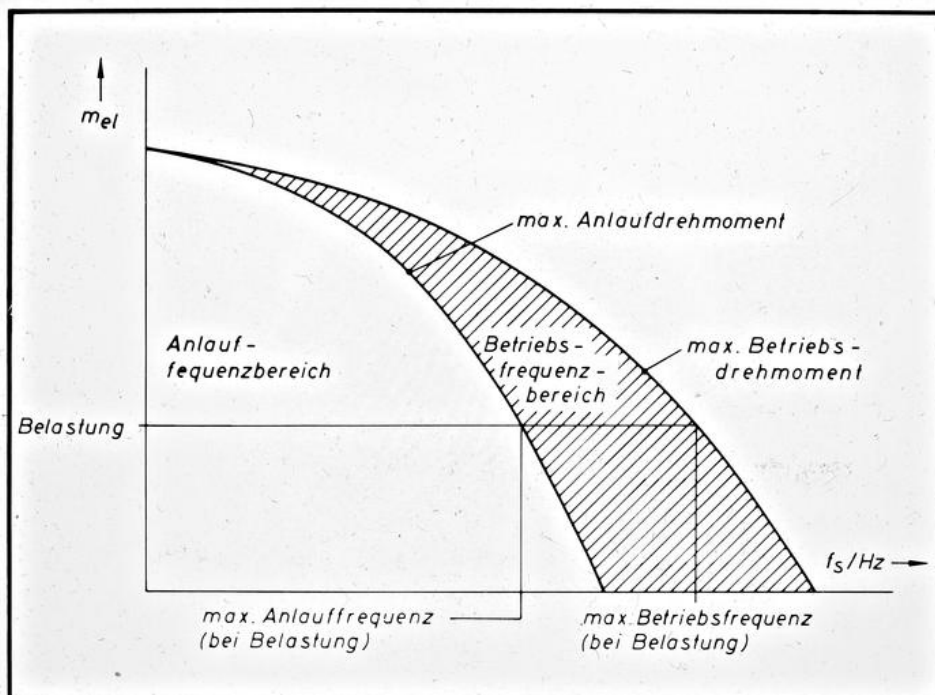
EW THD Zur Definition der Anlauf- und Betriebswerte 2/3.28 von Schrittmotoren
