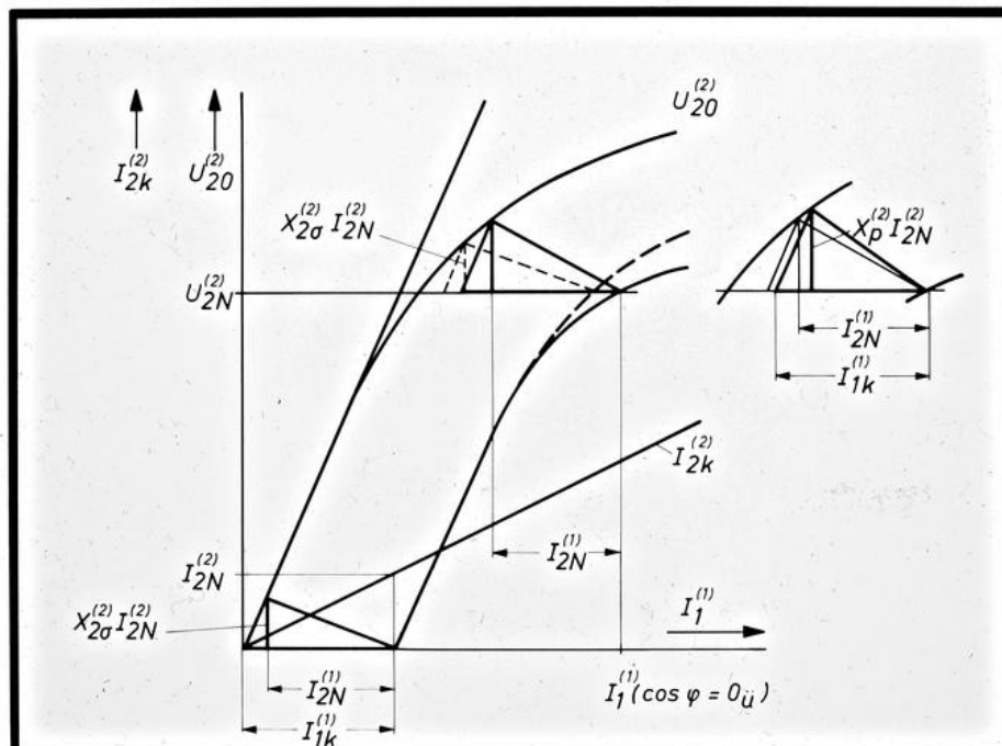
EW THD Das Potierdreieck der Synchronmaschine 1/9.9
