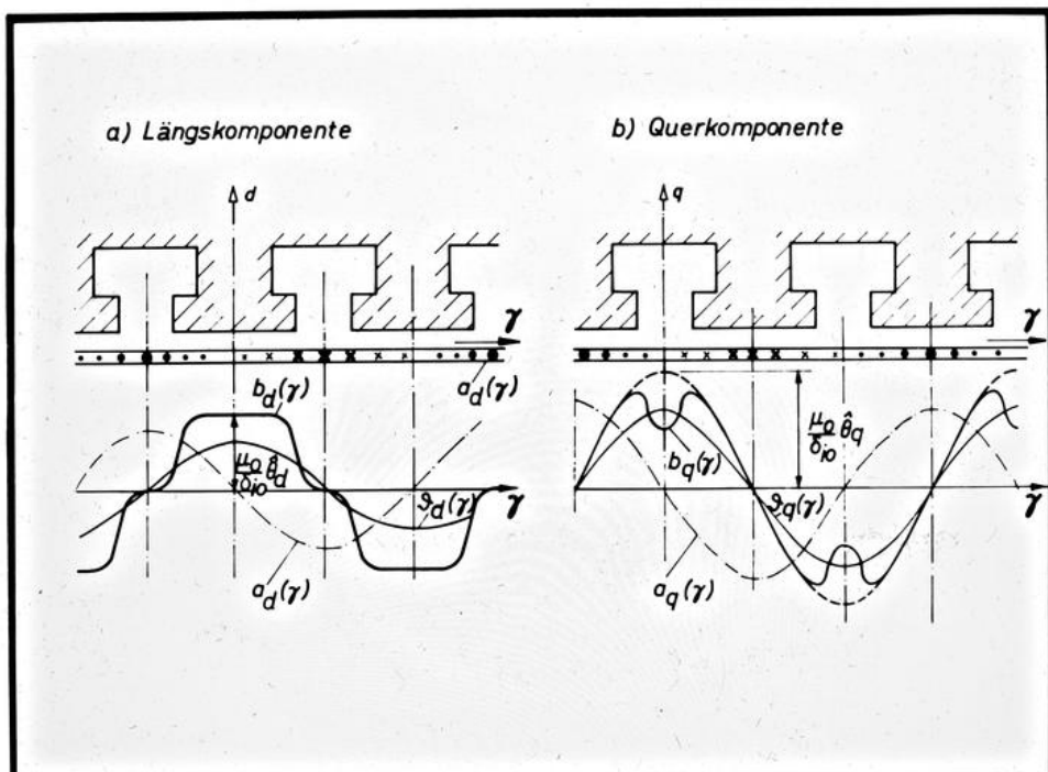
EW THD Induktionsverteilungen der Komponenten der Durchflutungsgrundwelle 1/5.14
