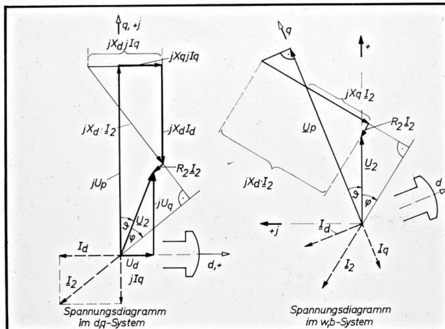
EW THD Zeigerdiagramm der Synchron-Schenkelpolmaschine, Generatorbetrieb, übererregt 1/9.1
