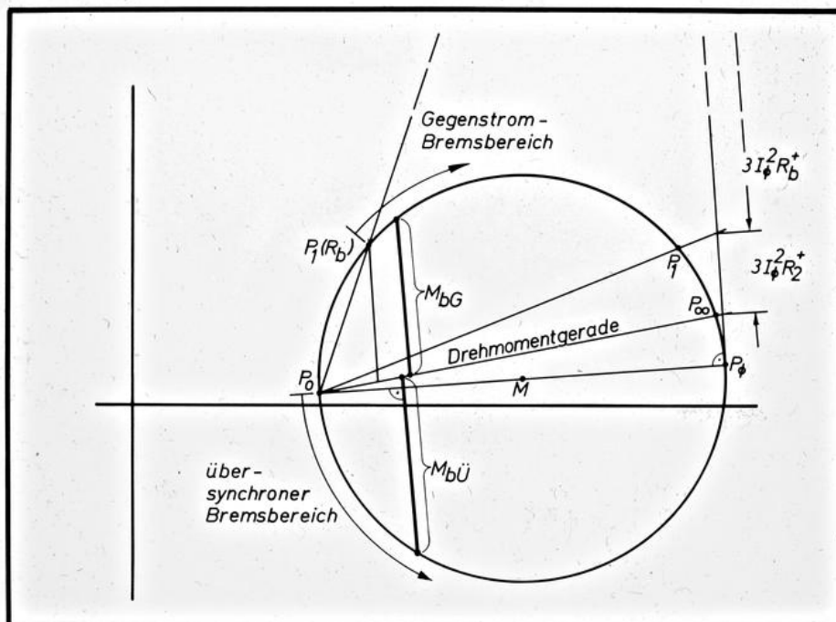
EW THD Die Bremsbereiche im Ossanna-Kreis
