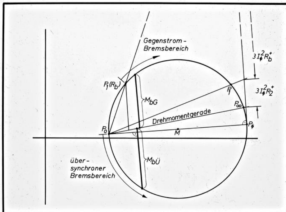
EW THD Die Bremsbereiche im Ossanna-Kreis
