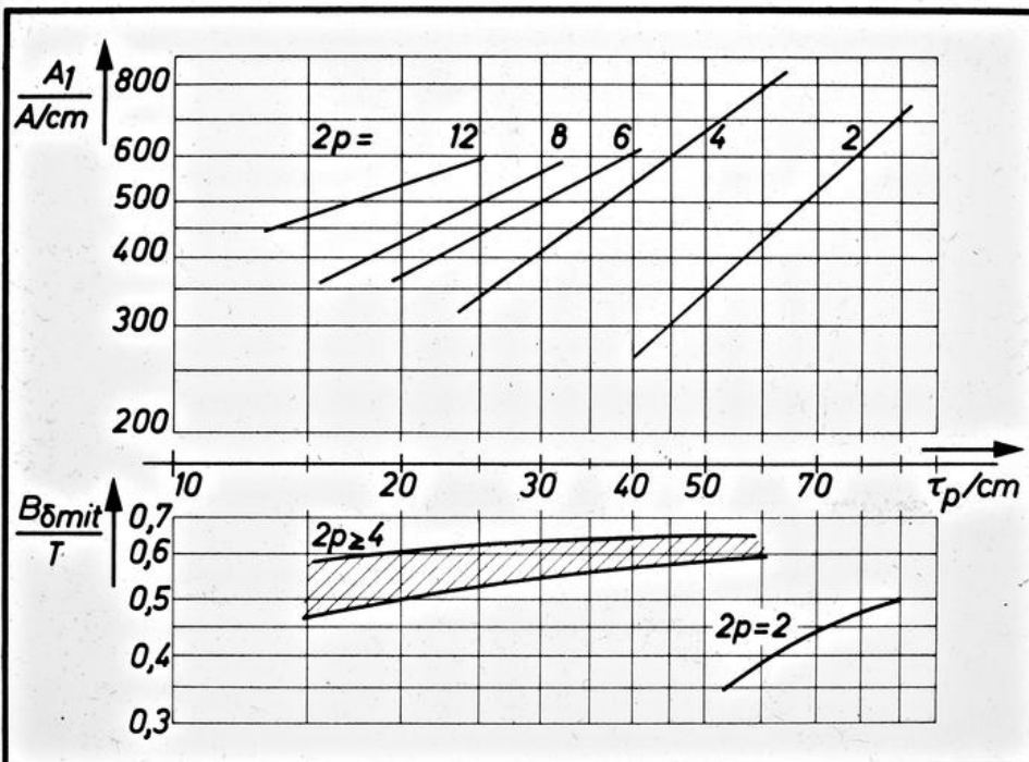
EW Strombelag A_1 und mittl. Luftspaltinduktion B_{\delta mit} 2/1.9 THD in Abhängigkeit v. der Polteilung \tau_p bei Asynchronm.
