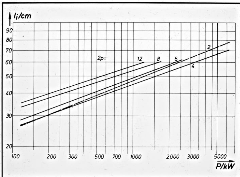
EW THD Ideelle Ankerlänge l_i in Abhängigkeit von der Nennleistung bei Asynchronmaschinen 2/1.6
