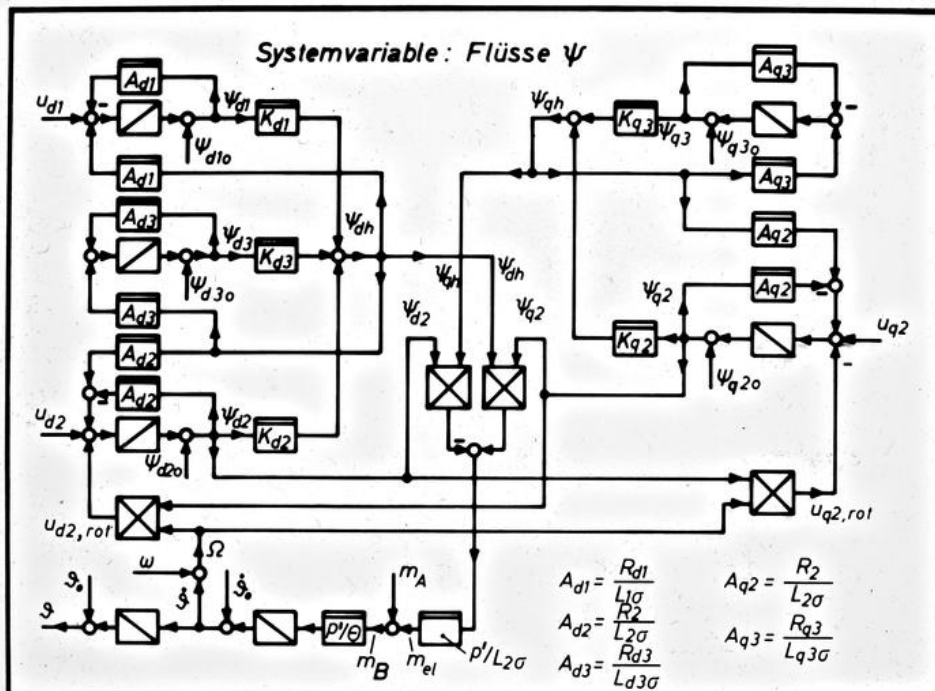
EW Strukturbild der transformierten Synchronmaschine im läuferbezogenen d,q-System
